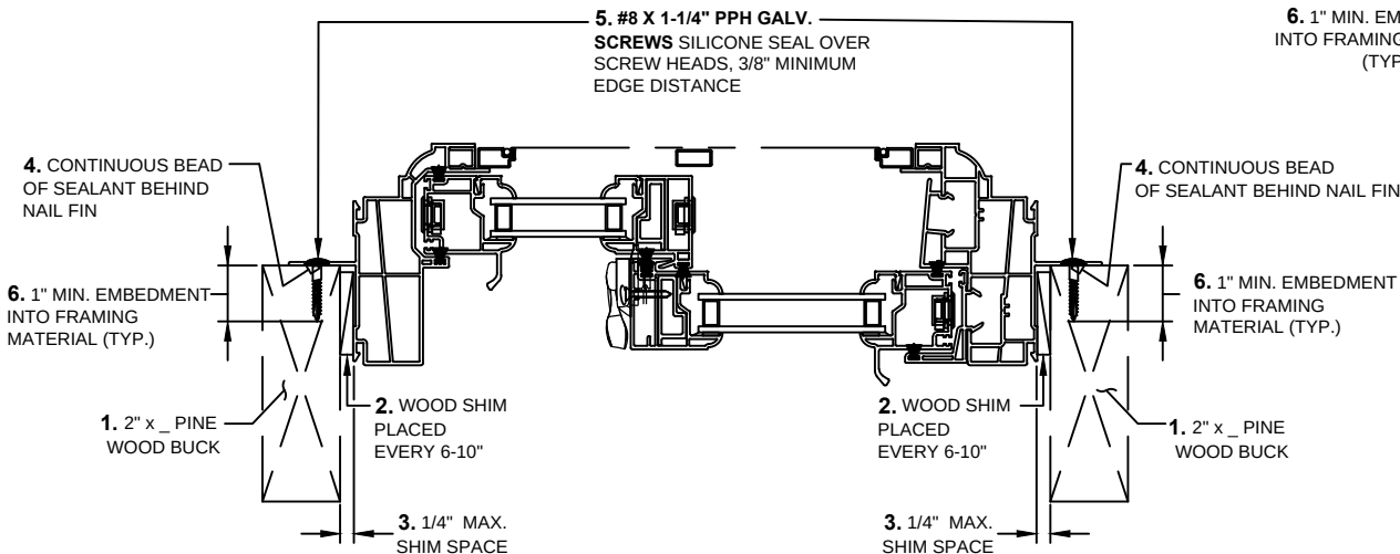
SIDE JAMB (TYP.)
